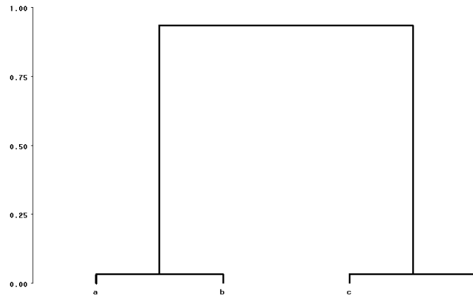
FIGURE 2.2 – Dendrogramme correspondant à la CAH sur les individus a, b, c et d
