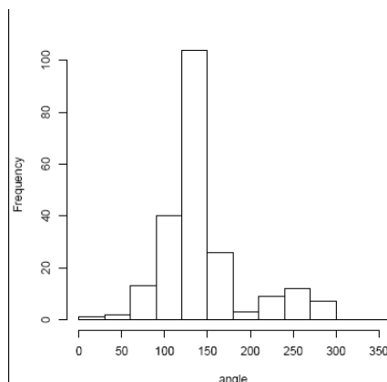
FIGURE 4.4 – Jeu de données (gauche) et histogramme des angles (droite)
