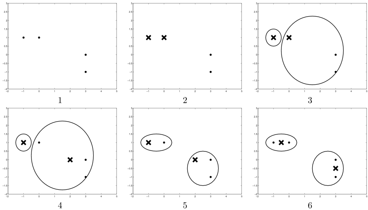
FIGURE 2.1 – Une illustration de l’algorithme K -means. (1) On dispose de 4 points à classer en deux classes. (2) À l’initialisation, deux de ces points sont choisis comme centres de classe. (3) Deux classes sont créées en regroupant les autres points en fonction du centre de classe le plus proche. (4) On définit les nouveaux centres de classe comme étant le barycentre des classes nouvellement créées. (5) On regroupe à nouveau les points. (6) On définit les nouveaux centres de classes. A l’étape suivante rien ne change, l’algorithme a convergé.
