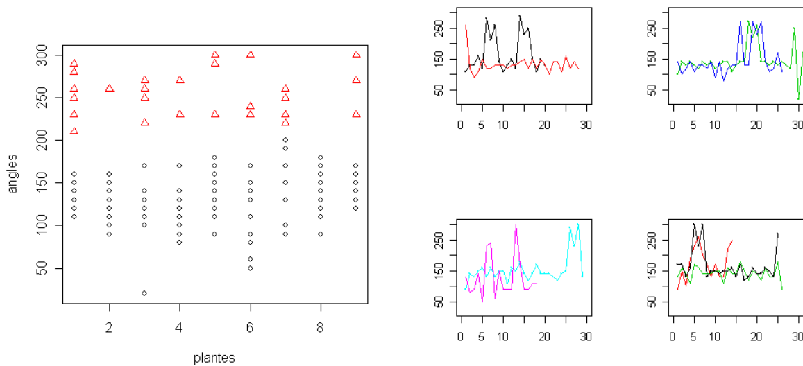
FIGURE 4.6 – Classification à 2 groupes : classification des angles en fonction de la plante (à gauche) et profils des angles par plante (à droite).
