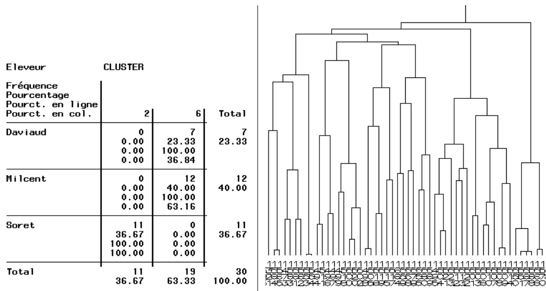
FIGURE 4.3 – Gauche : Comparaison classe / élevage d’origine pour les Noires de Challans. Droite : Sous-partie du dendrogramme représentant la classe contenant 19 Noires de Challans et 30 Coucous de Rennes.
